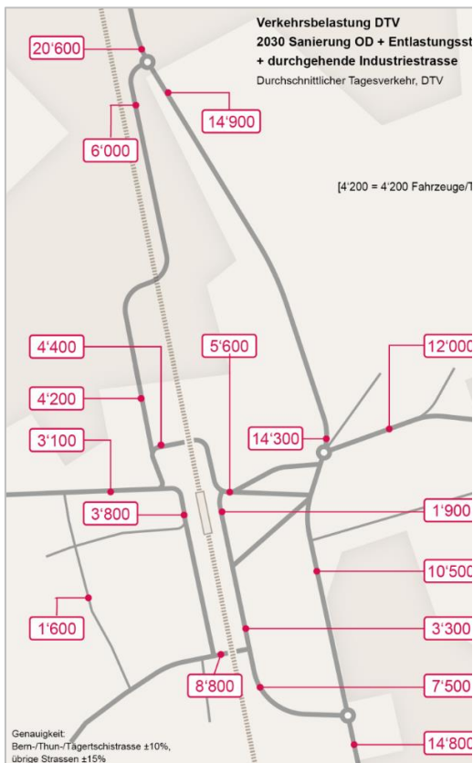
Verkehrsbelastung DTV 2030 mit Sanierung der Ortsdurchfahrt + Entlastungsstrasse Nord + durchgehende Industriestrasse
