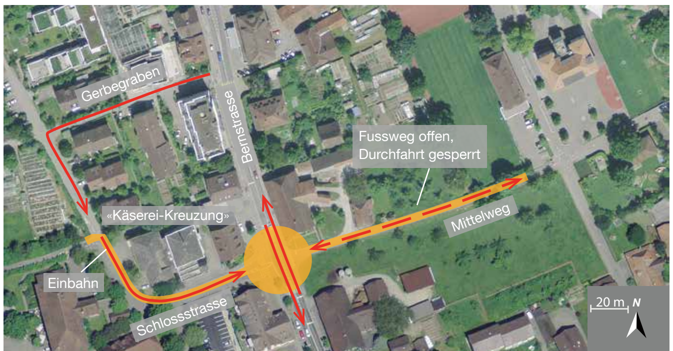
Übersicht über den Baustellenbereich (orange) und die Verkehrsführung (rot). (Luftbild: Swisstopo, 2016)
