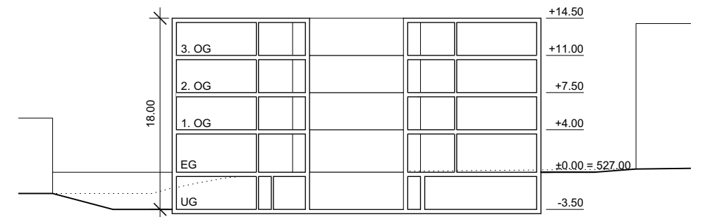
Schnitt B-B
